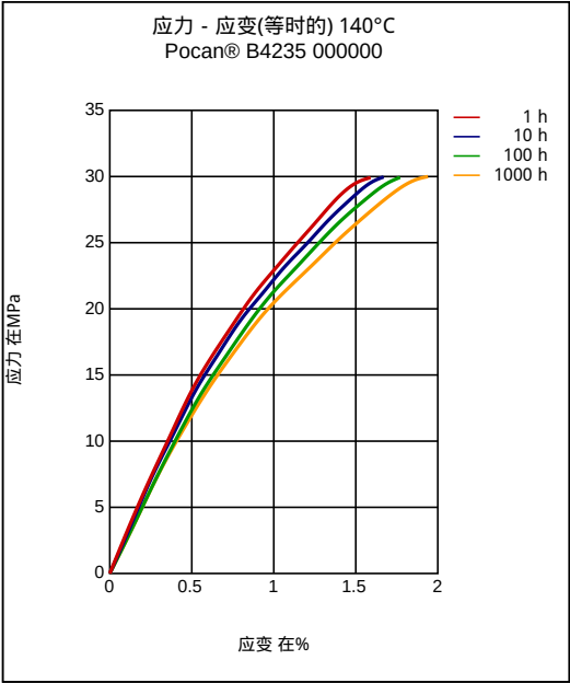
应力 - 应变(等时的) 140°C
